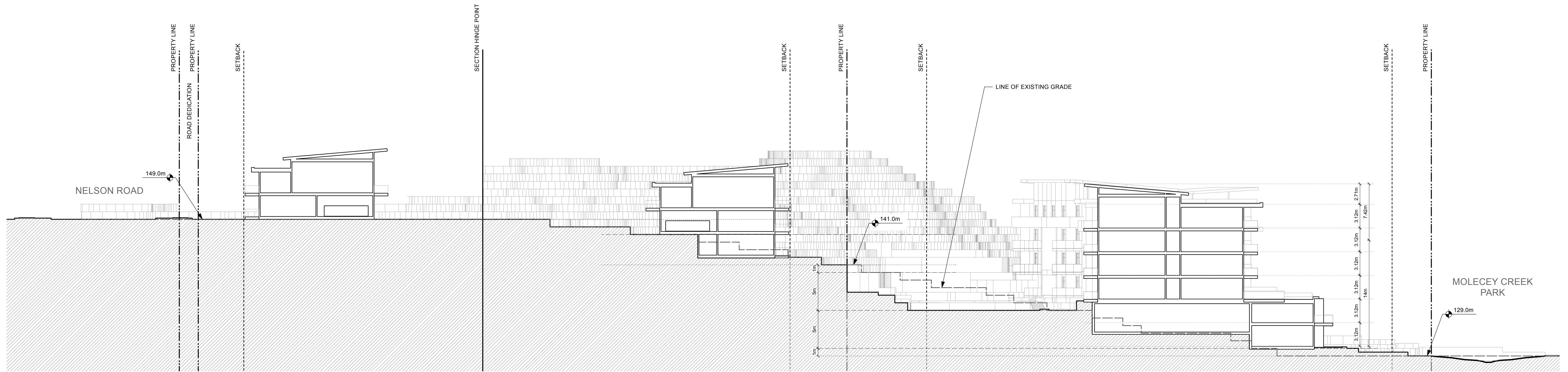
2 Site Section A400 Scale: 1:250
