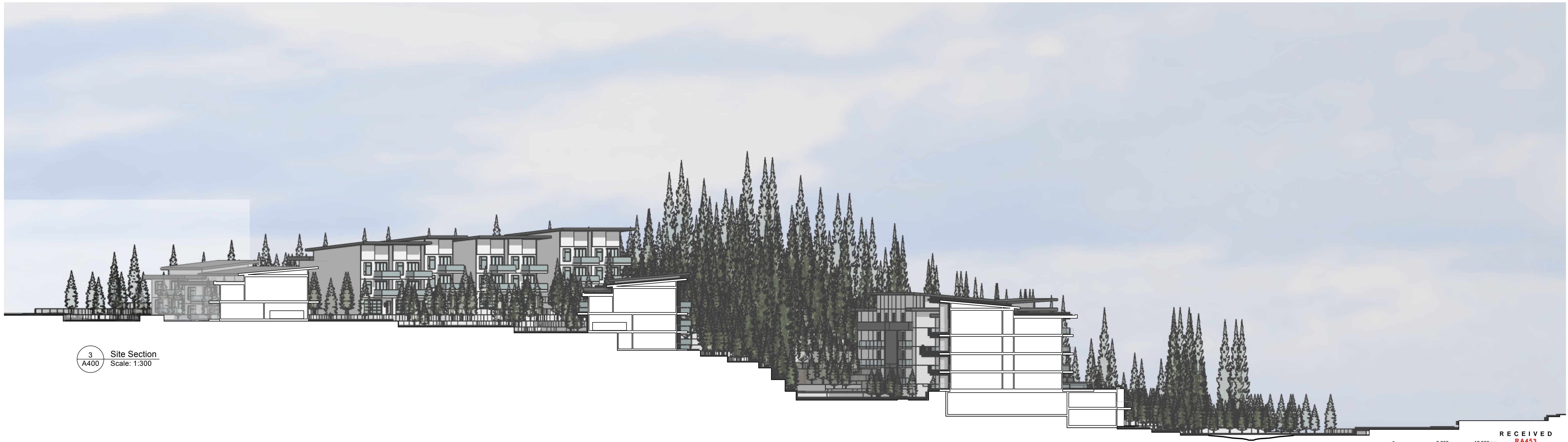
2 Site Section A400 Scale: 1:250
